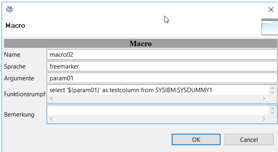
Abbildung 4-8 Bearbeitung eines Makros in der GUI
