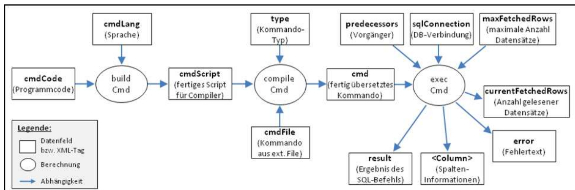
Abbildung 4-7 Aufbau eines Kommando
