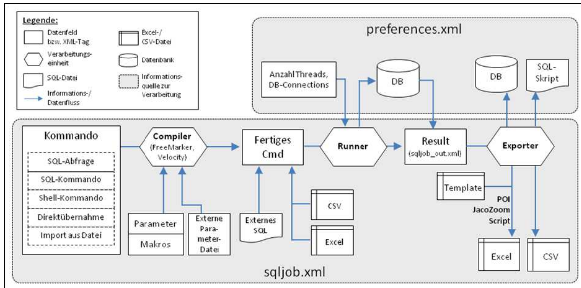
Abbildung 4-5 Architektur des SqlSurfers
